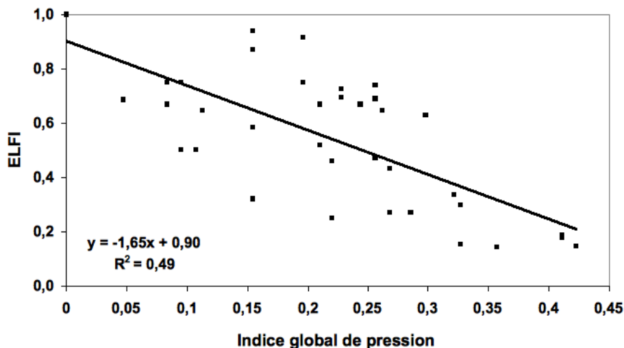
Figure 2 : Régression linéaire entre les pressions (indice global) et l'état mesuré par l'indicateur poisson ELFI (valeur des EQR entre 0 et 1)
